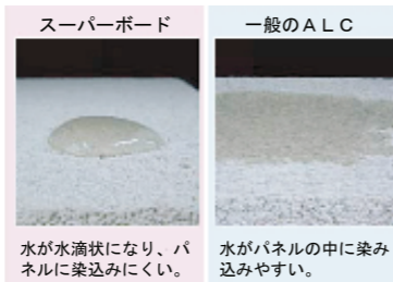
撥水試験状況 (社内試験)
